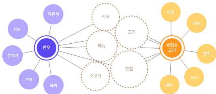
분석단어별연관어순위
